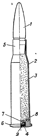
Рис. 71. Боевой патрон:
