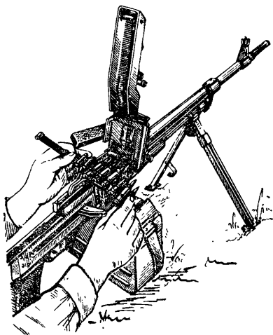
Рис. 81. Вкладывание ленты в при- смник
