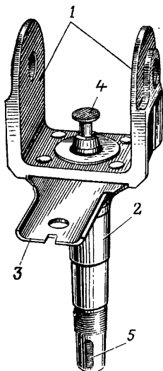
Рис. 59. Вертлюг:
