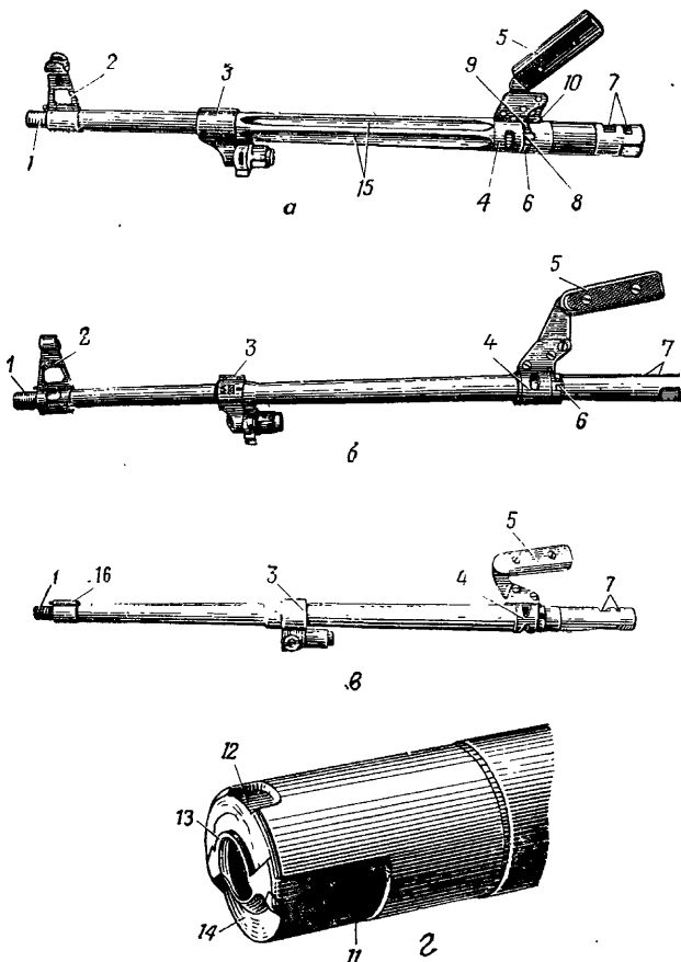
Рис. 24. Ствол:
