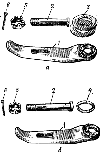
Рис. 58. Зажимы ног:
