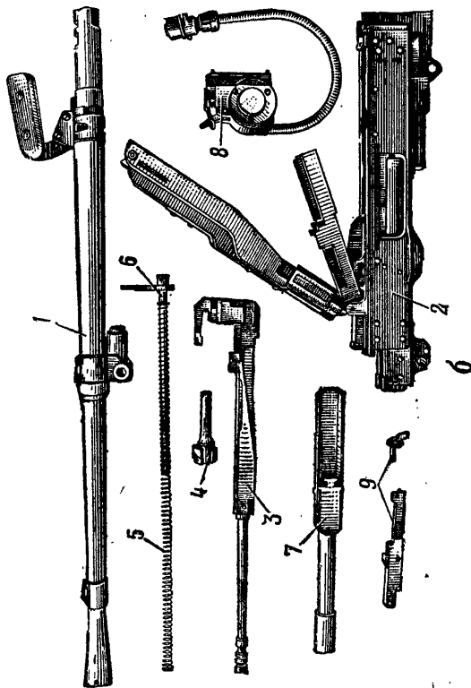
Рис. 2. Основные части и механизмы пулеметов Калашникова:
