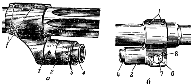
Рис. 26. Газовая камера:
