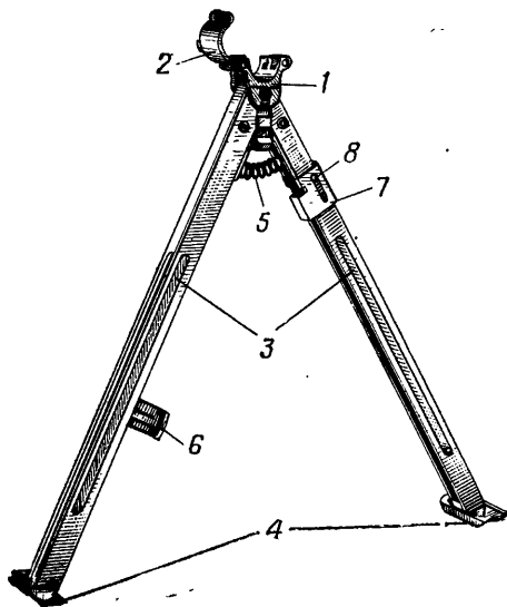
Рис. 37. Сошка:
