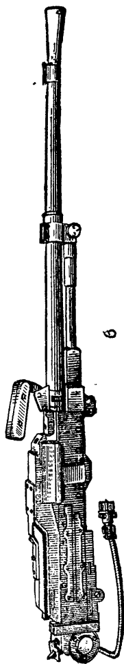
Рис. 1. Общий вид пулеметов Калашникова: а — пулемет ПКМ; б — пулемет ПКС; в — пулемет ПКТ
