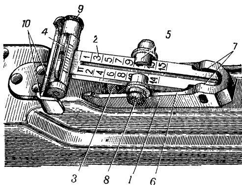
Рис. 45. Прицел:
