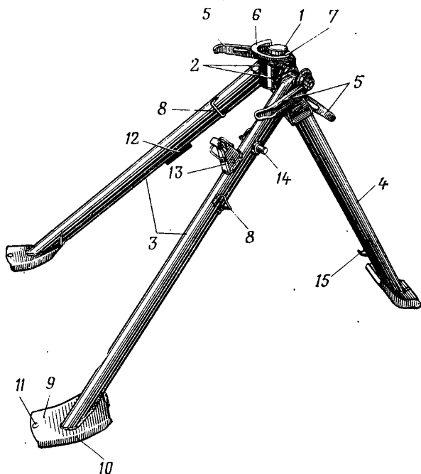
Рис. 55. Основание станка:
