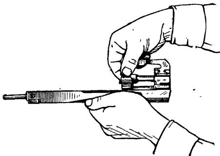
Рис. 8. Отделение затвора от затворной рамы
