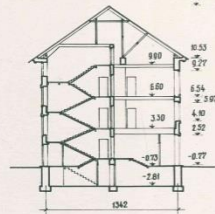
Разрез
