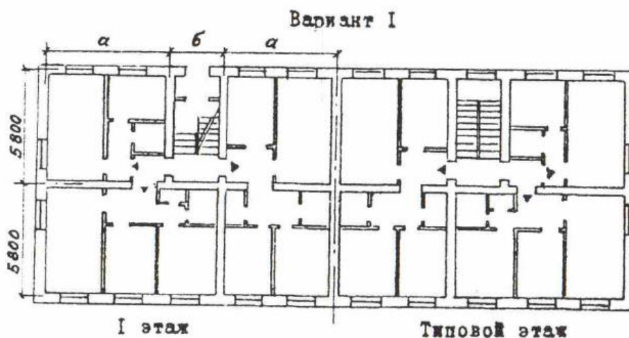
Строительные размеры здания.
