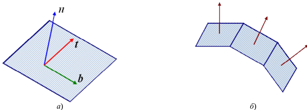
Рис. 31. Неискаженный вектор нормали к грани определяется в касательном пространстве (a) и равен (0, 0, 1)
