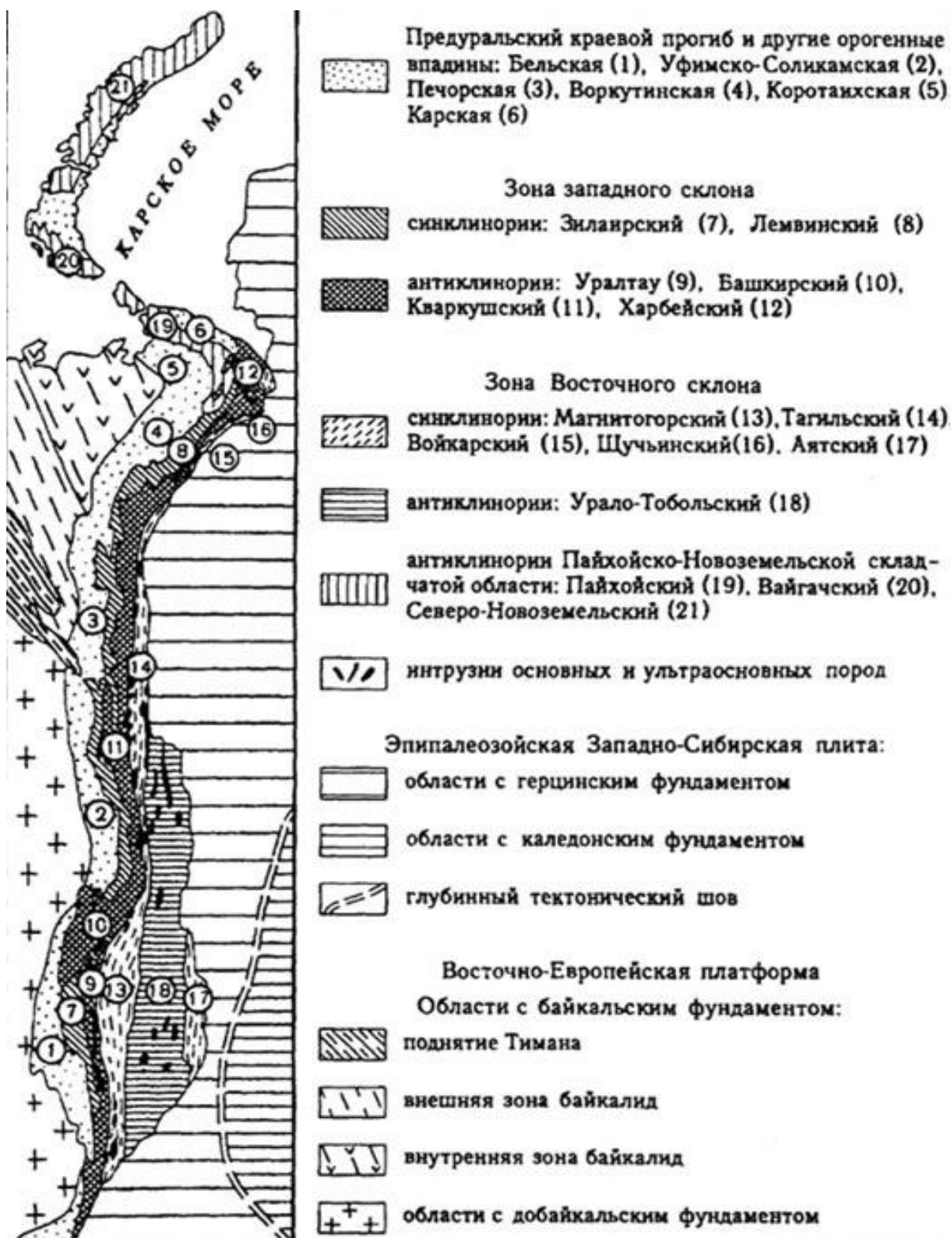
Тектоническая схема Урала
